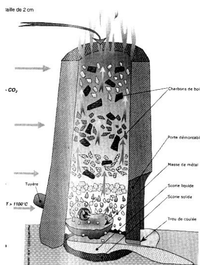
Figure 8 : Schéma d'un four à scorie écoulee (DAO Paul Merluzzo)
