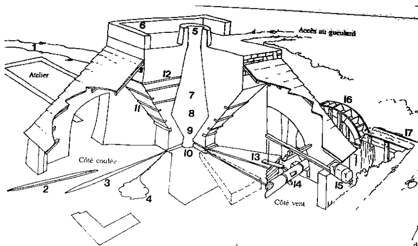
Figure 11 : Schéma d'un haut fourneau du XVIII e siècle (tiré d'Andrieux 1988)
