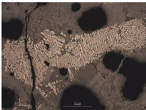
Figure 32 : Battiture tombée dans la scorie liquide au fond du foyer de forge. Elle a été figée alors qu'elle était en cours de fusion
