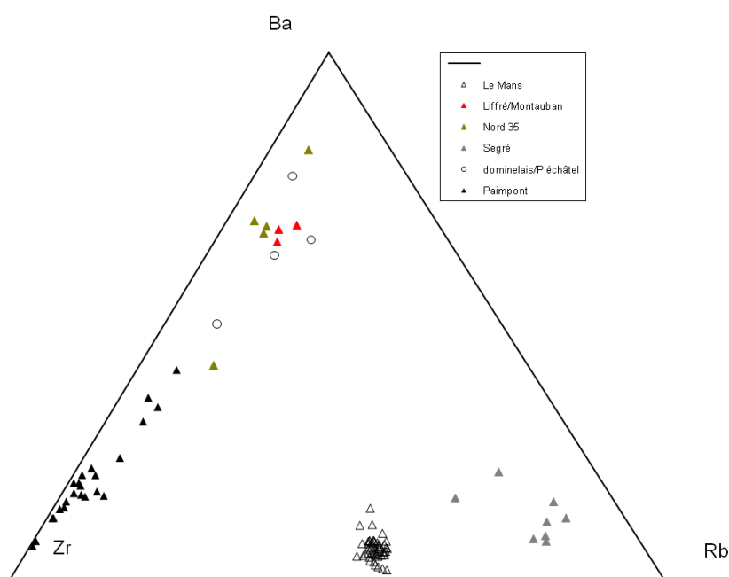
Figure 34 : Diagramme chimique montrant des différences entre les scories de réduction en bas fourneaux provenant de différentes régions du Massif armoricain. Il faut remarquer que certaines zones sont difficilement différenciables
