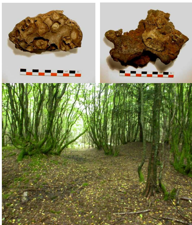
Figure 24 : Exemples de scories spongieuses provenant de sites situés en forêt de Paimpont. Leur accumulation forme de gros ferriers
